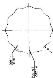
CORTE 4-4 12 ESTRIAS REPARTIDAS EN EL ENVASE COMO SE MUESTRA
